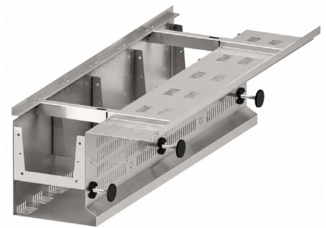
DRAINTEC Sockelrinne mit der Auskrägung
